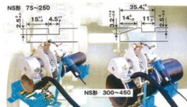
オートパイプカッター OP-3 NS仕様 75-450用
