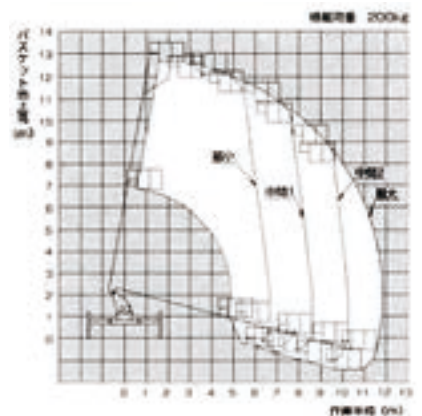
※上図は、HPPバケット仕様のもので、
