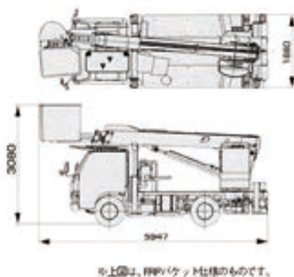
※上図は、HPPバケット仕様のもので、
